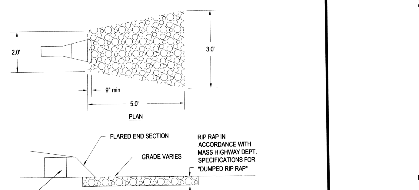
F.E.S. W/ RIP RAP
