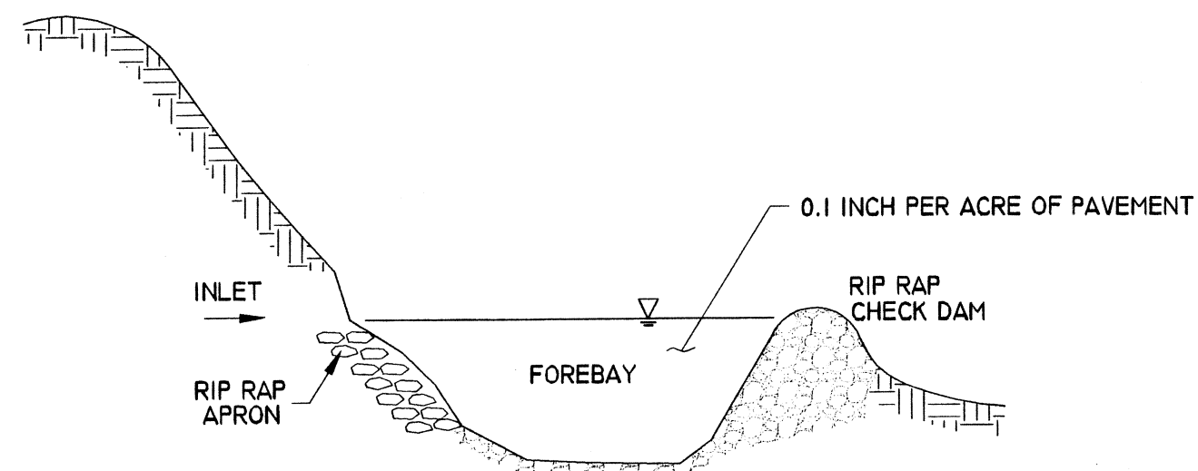
SEDIMENT FOREBAY - SECTION
